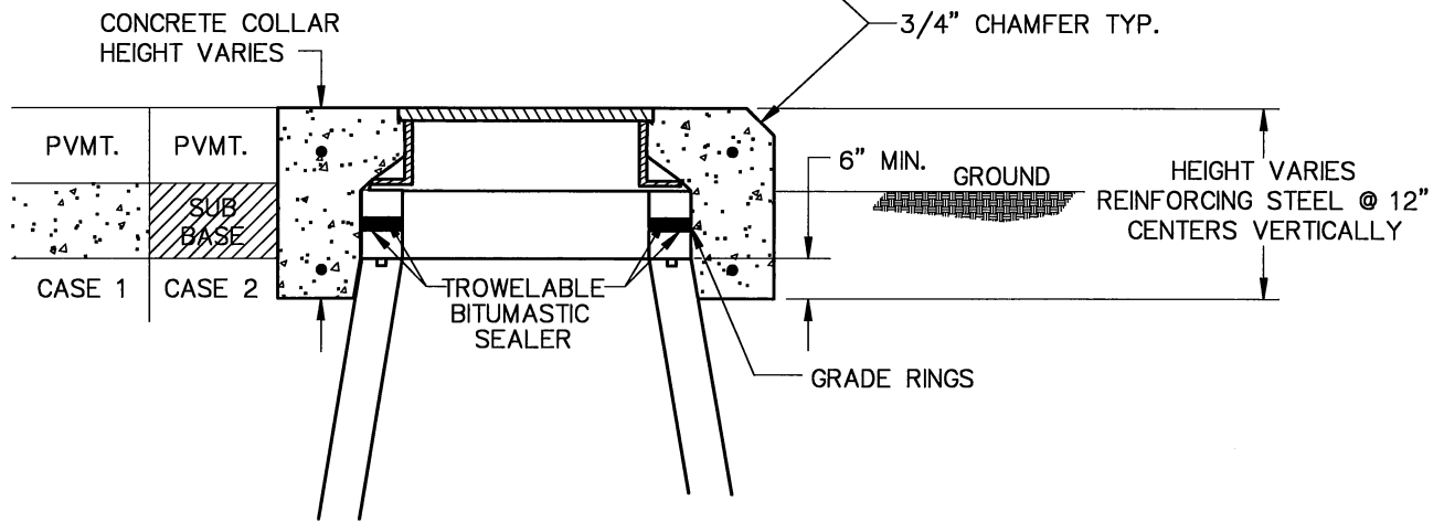
SECTION A-A
