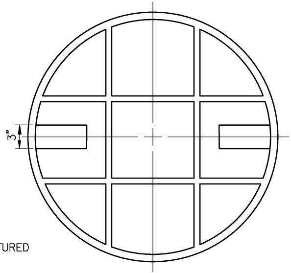
LID - BOTTOM VIEW
